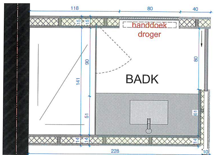
3E VERDIEPING - DETAIL BADKAMER Schaal: 1/20
